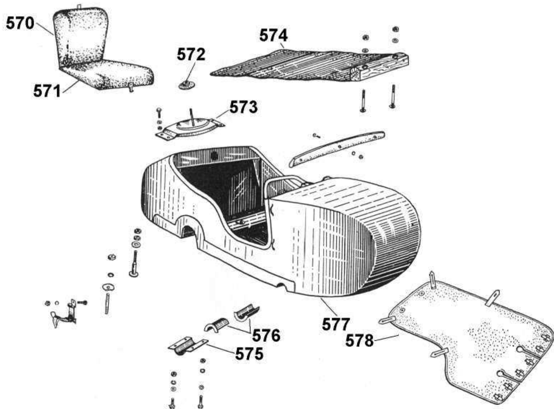
Рис. 33. Кузов коляски.
