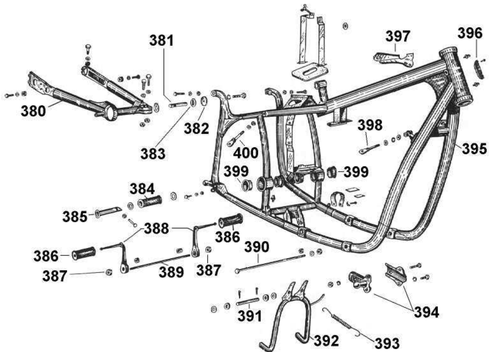
Рис. 19. Рамы, подставка, подножки.
