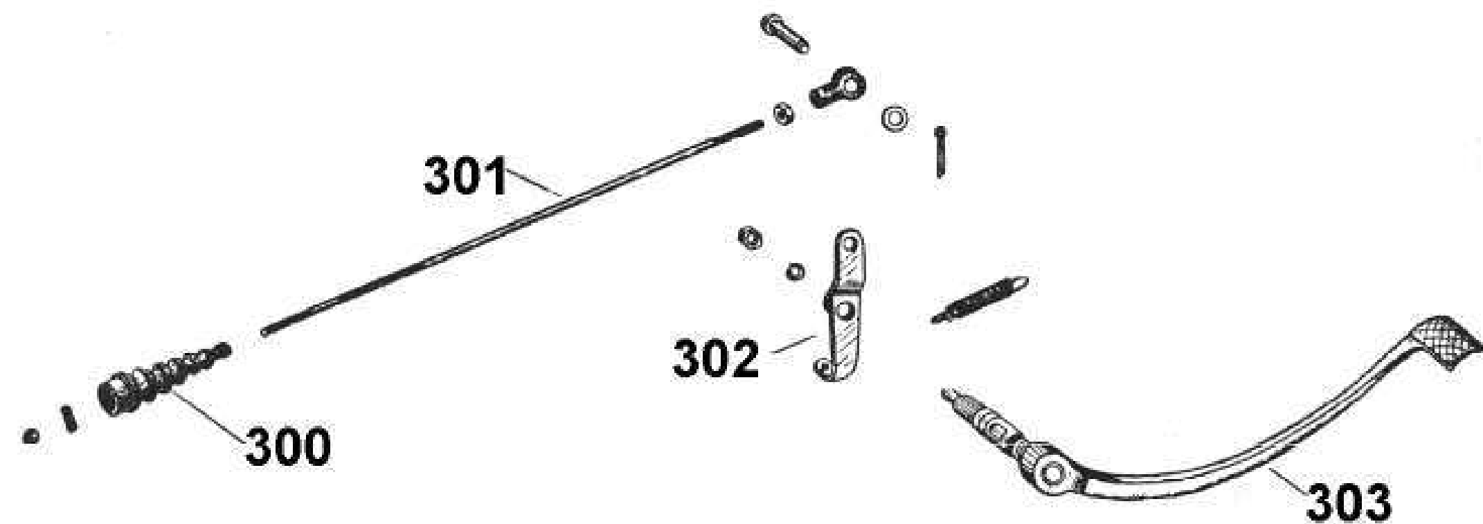
Рис. 25. Привод заднего тормоза.
