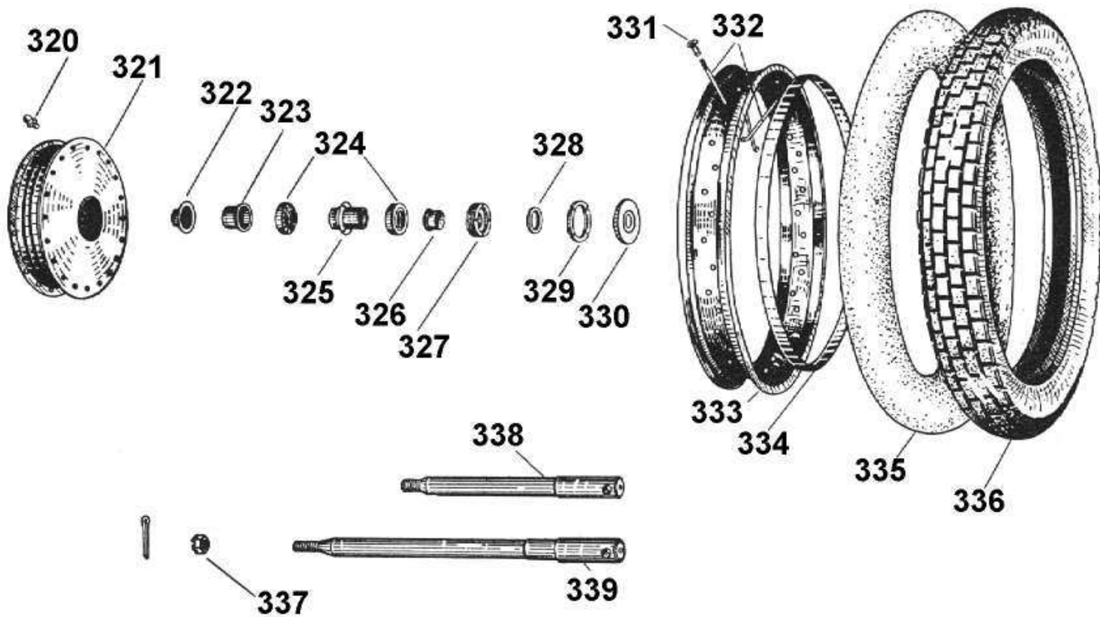
Рис. 16. Колесо со ступицей.
